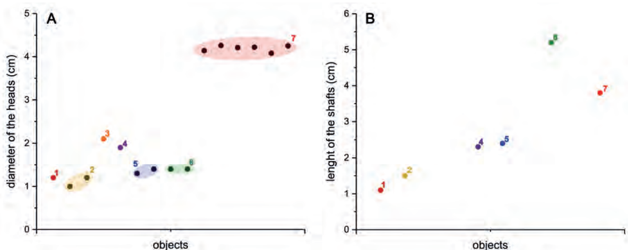
Figure 6: Diagrams of the diameter of the rivet heads (A), highlighting the uniqueness of the Figueiredo das Donas group, and the size of the shafts (B). 1. Alegrios; 2. Columbeira; 3. Cabeço do Castro de São Romão; 4. Moinho de Golas; 5. Monte do Trigo; 6. Pragança; 7. Figueiredo das Donas.
