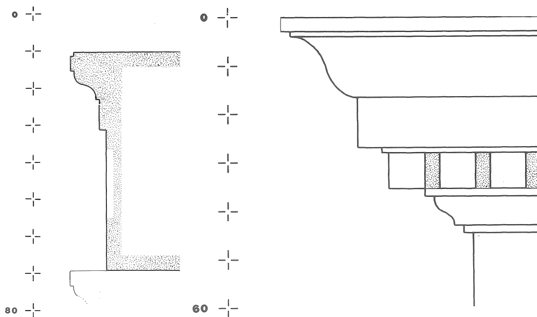
FIGURA 79. Secció del fris de l'arc.
