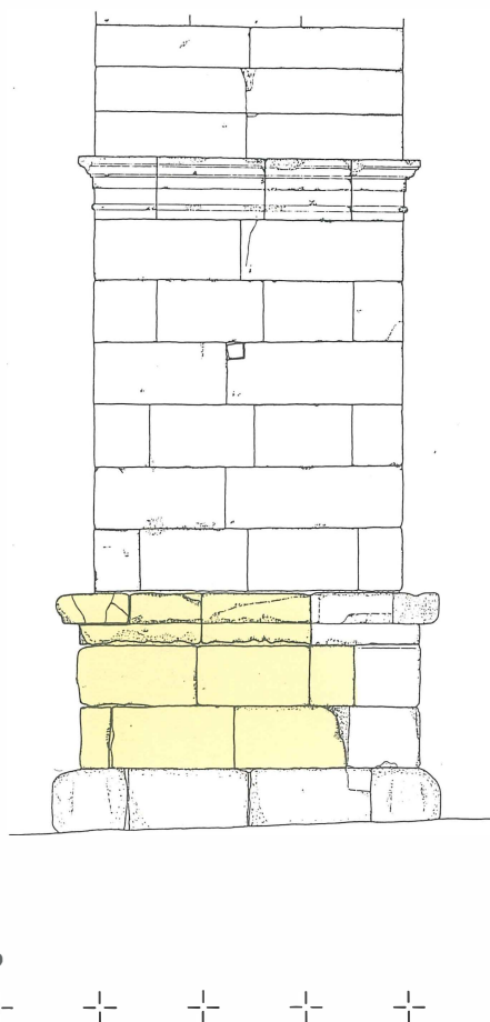
LÀMINA XII. Arc de Berà. Alçat del parament intern del pilar occidental amb indicació dels elements corresponents a la restauració de 1788.
