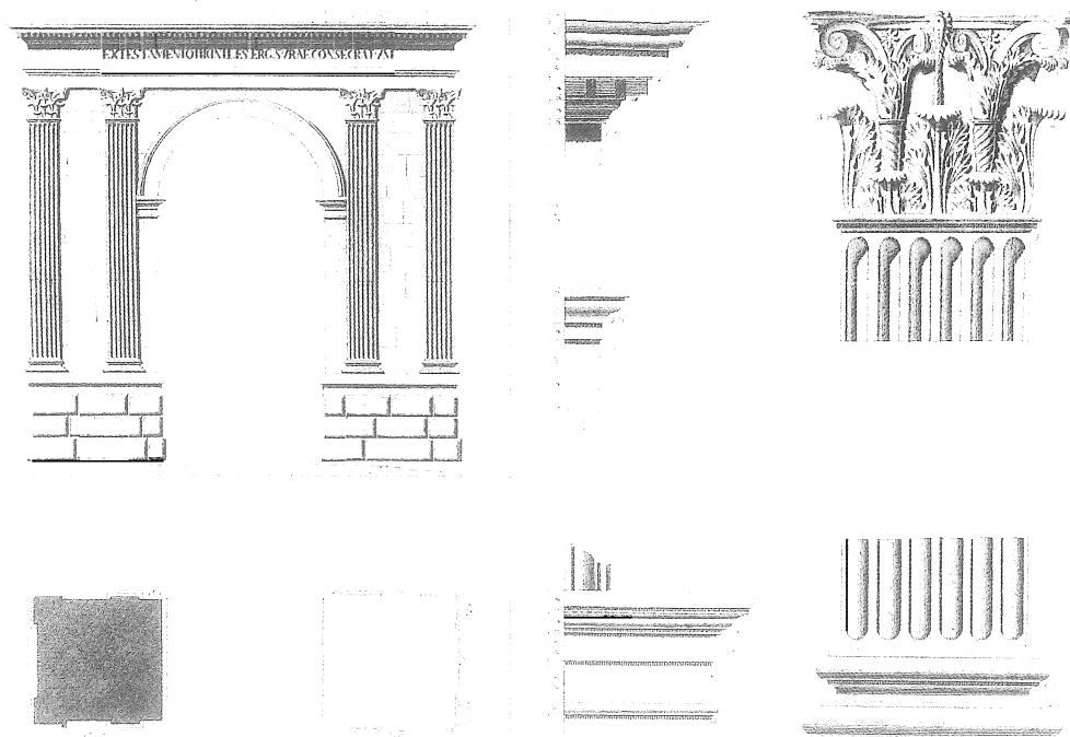
FIGURA 18. Aiguafort amb l'alçat, la planta i diversos detalls arquitectònics de l'arc, publicat per Alexandre de Laborde (fotografia Biblioteca de Catalunya).
