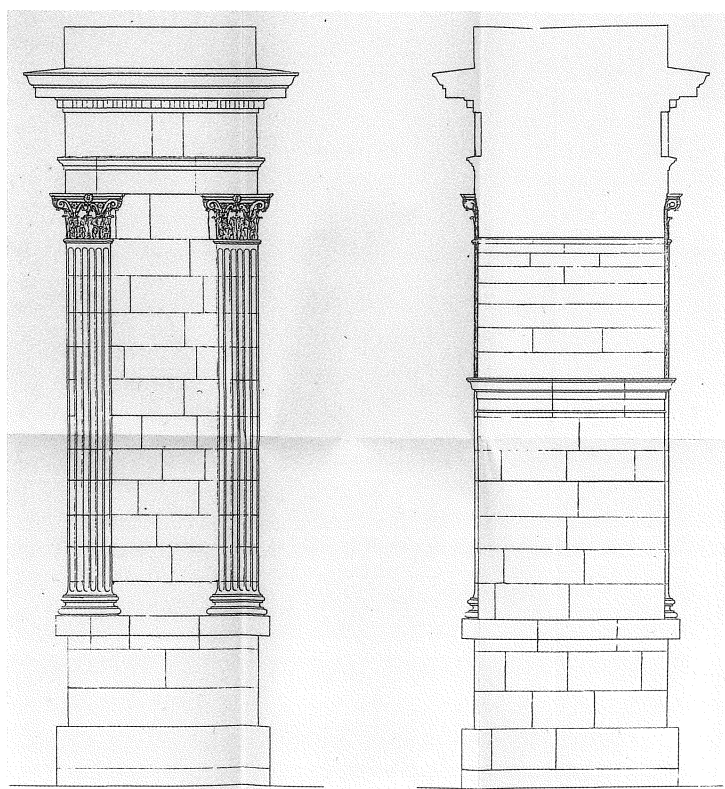
FIGURA 40. Alçat reconstructiu d'un dels laterals i secció del monument, realitzats per Reventós i Rubió l'any 1931 (fotografia Museu Nacional Arqueològic de Tarragona [Pasqual Serres], núm. neg.: 856/5).
