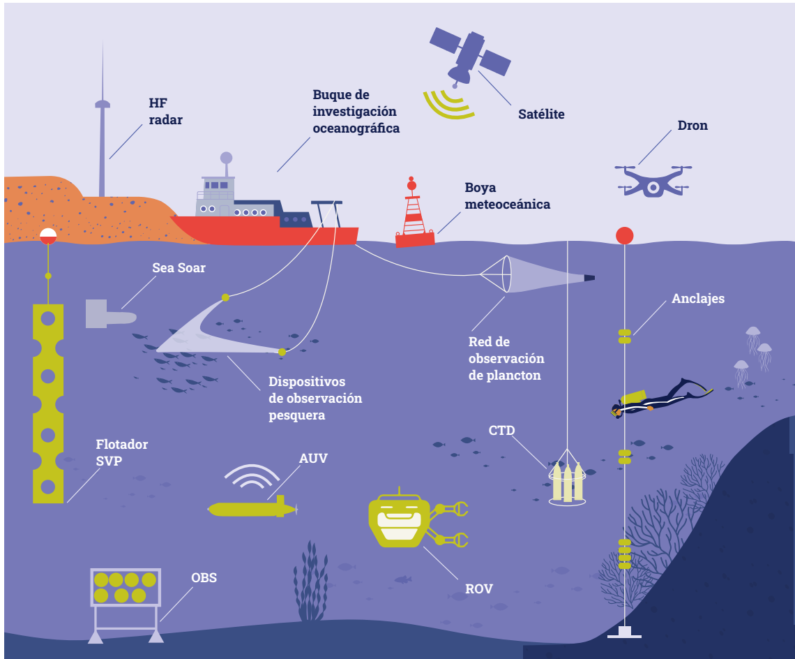
Gráfico 12 Esquema de un sistema de observación oceanográfica multiparamétrica con los diferentes tipos de instrumentos y estrategias de muestreo
