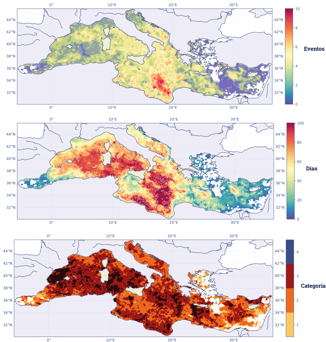
Gráfico 6 Características de la ola de calor marina en la cuenca del Mediterráneo en el verano de 2003
