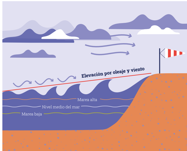
Gráfico 7 Componentes que contribuyen a las variaciones del nivel del mar durante un temporal costero
