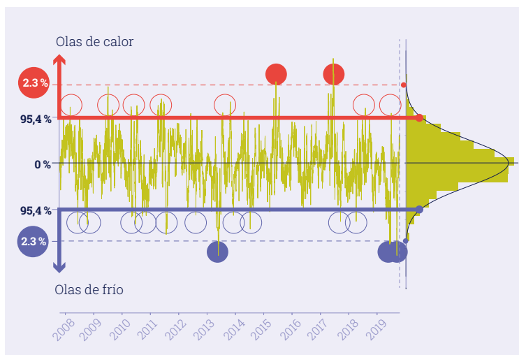
Gráfico 5 Detección de olas de calor marina en el área de las islas Columbretes, a partir de una serie temporal de temperatura de la superficie del mar [curva irregular]
