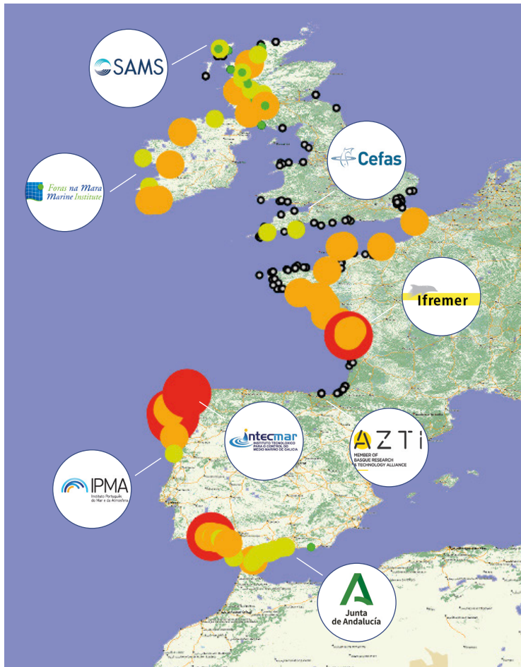
Gráfico 15 Mapa de proliferaciones de algas nocivas a nivel europeo de la especie Dinophysis acuminata (productora de toxina diarreica) durante septiembre de 2020
