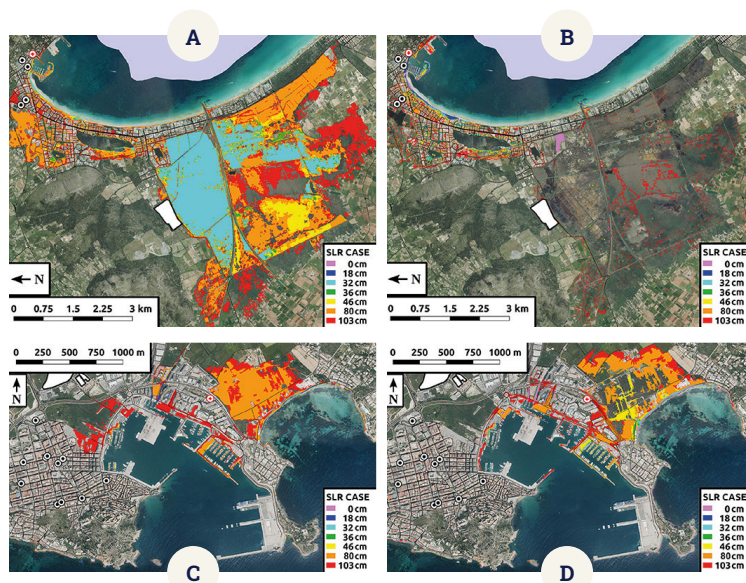
Gráfico 13 Extensión de las inundaciones permanentes y extremas, por distintas estimaciones de subida del nivel del mar, sobre el humedal de Alcúdia, Mallorca [A, B] y el puerto de Ibiza [C, D]
