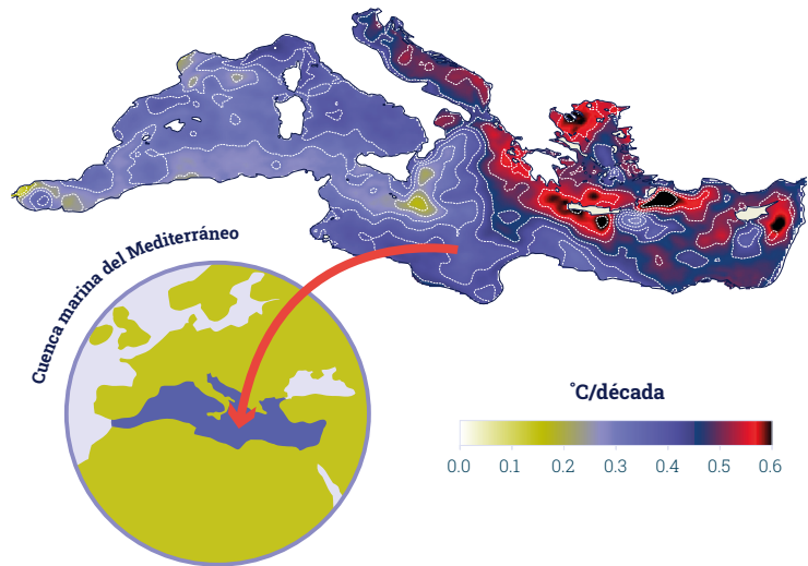
Gráfico 4 Calentamiento de la superficie de la cuenca marina del Mediterráneo en grados por década a partir de datos de satélite del periodo 1982-2022
