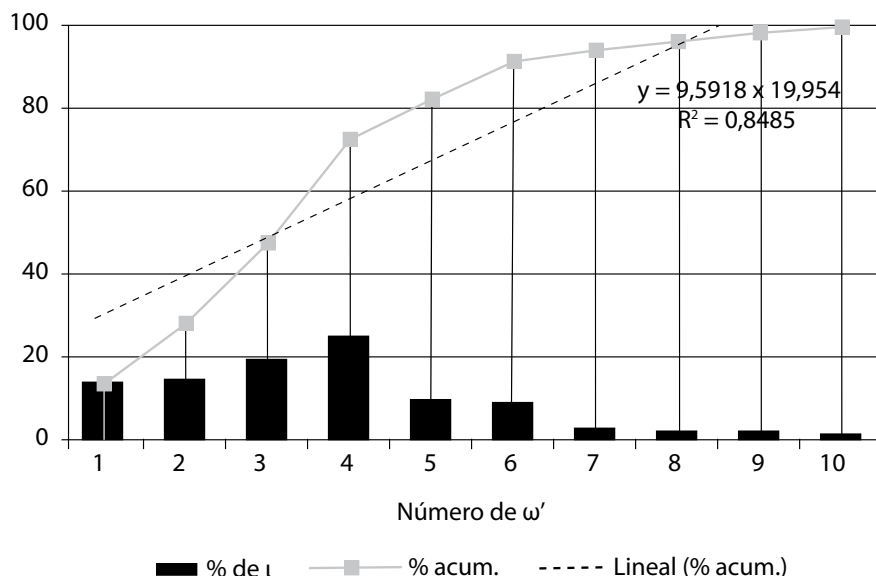
FIGURA 5. Proyección del porcentaje de t según el número de \omega' ; N (t)= 144; N ( \omega' )= 537.
