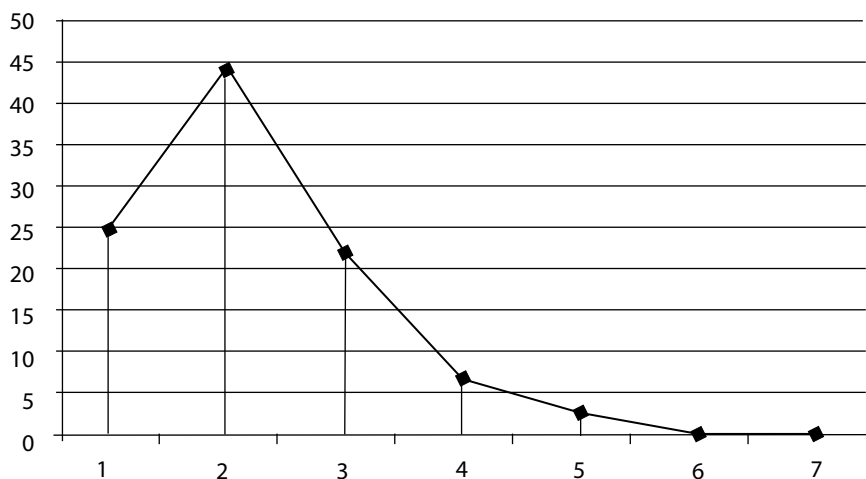
FIGURA 1. Porcentaje de \omega según número de \sigma
